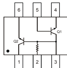
SOT26
